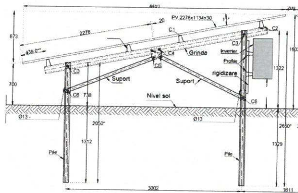
Figura 3. Detaliu montaj invertor
